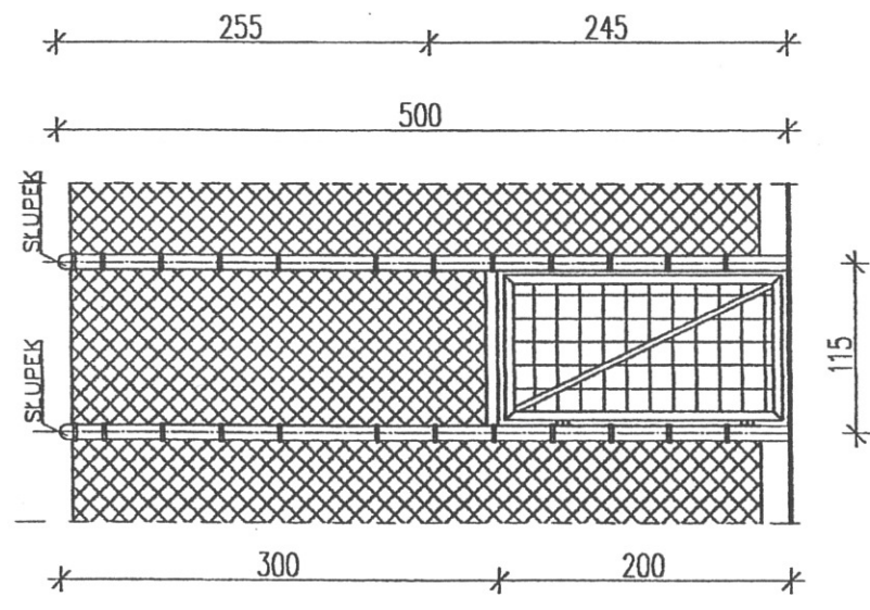
SCHEMAT FURTKI W OGRODZENIU SZT.1
